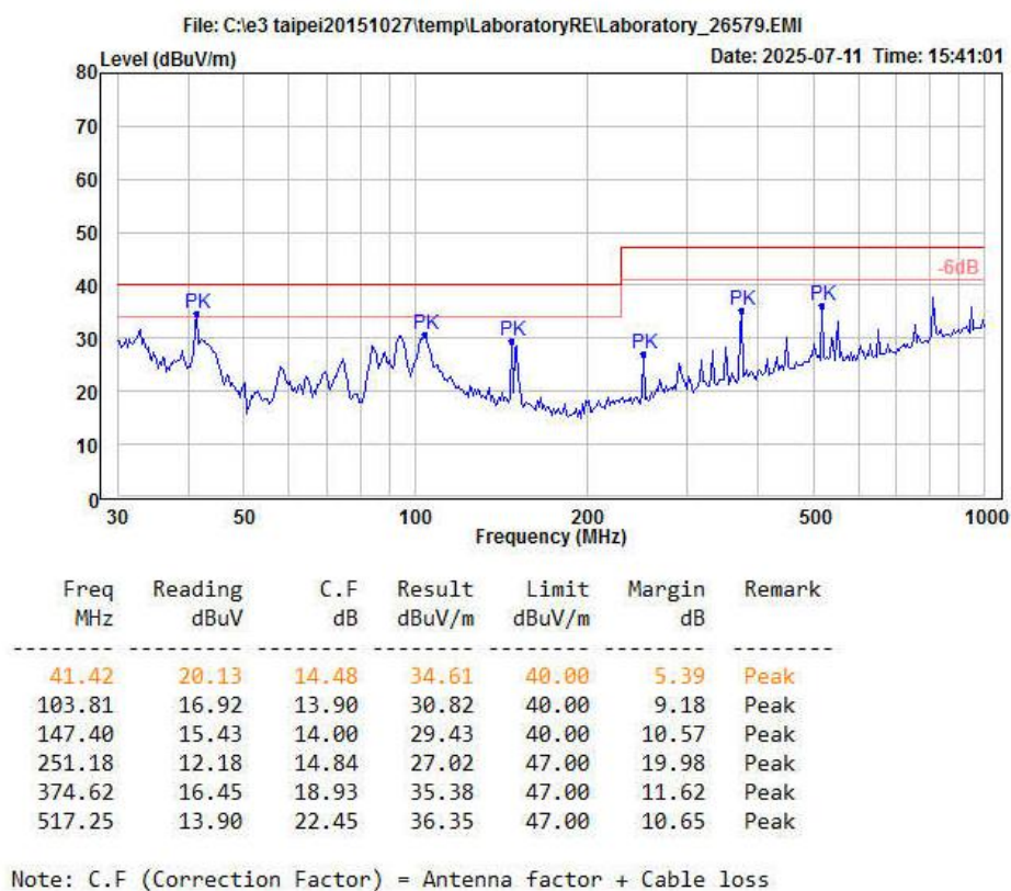
图 6-7 辐射测试垂直方向
