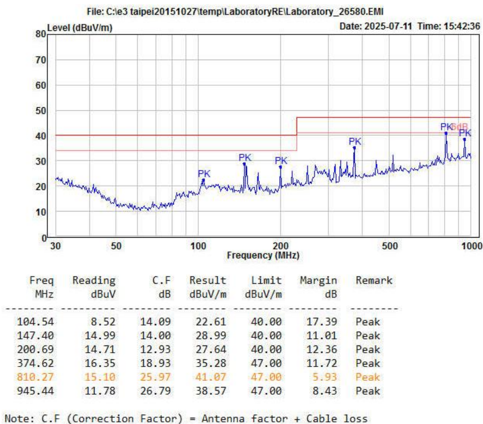
图 6-6 辐射测试水平方向
