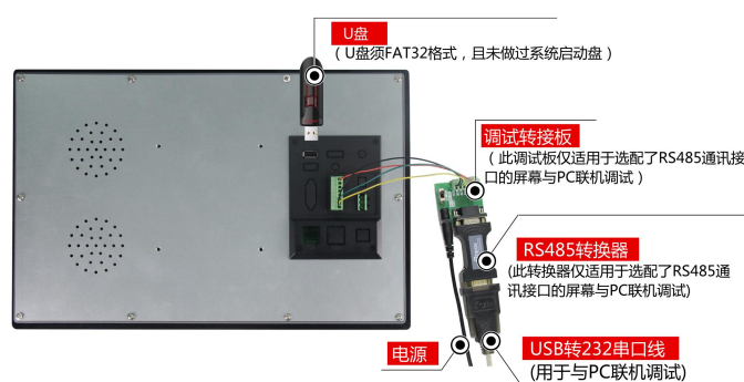
图 1-4 RS485 调试工具图
